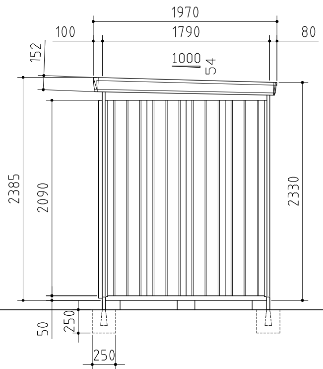
側面図
