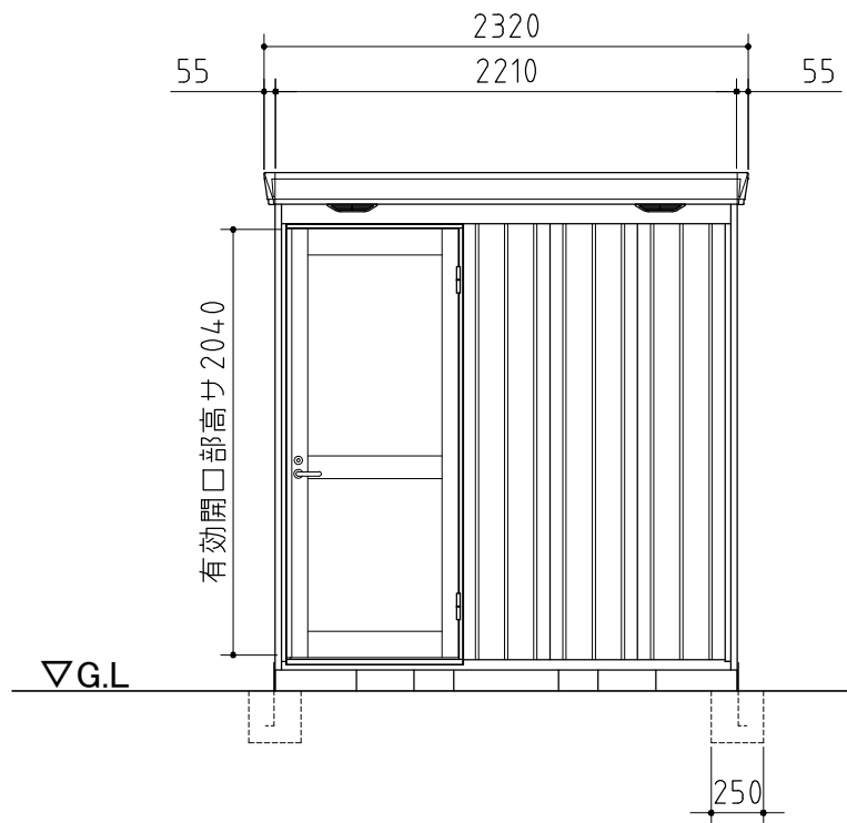
正面図
